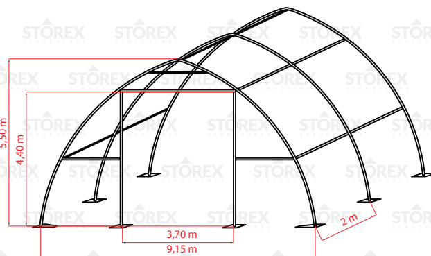
Частичный пространственный чертеж (показаны не все арки рамы)
