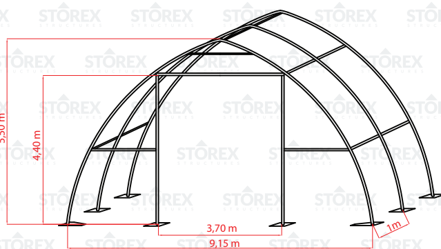
Частичный пространственный чертеж (показаны не все арки рамы)
