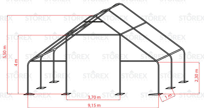
Частичный пространственный чертеж (показаны не все арки рамы)
