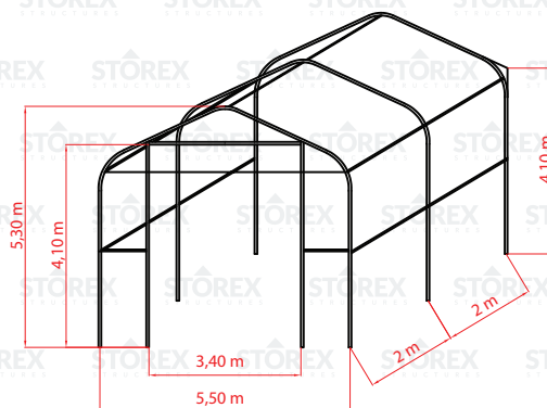
Частичный пространственный чертеж (показаны не все арки рамы)
